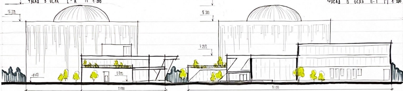
Разрез А-А М 1:200
